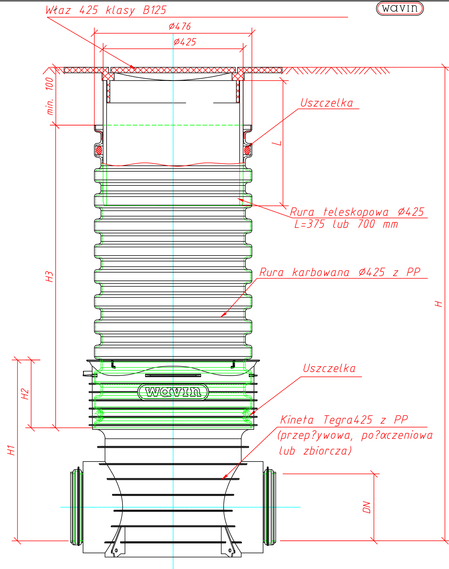
Studzienka inspekcyjna Tegra 425 z rurą teleskopową
